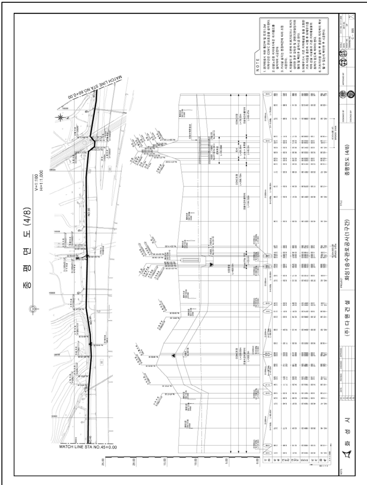
【그림 1.5】 화성1송수관로(1구간) 종평면도 (계속)
